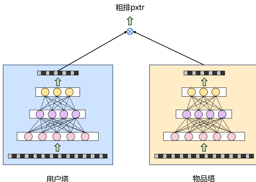
图 5.2: 粗排模型的双塔架构。
