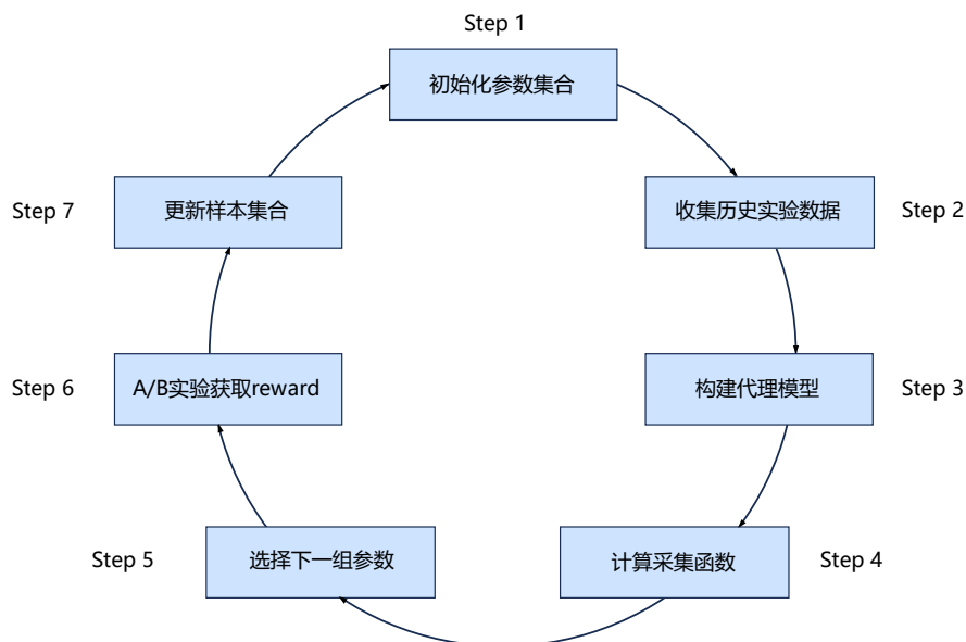
图 5.3: 推荐系统中贝叶斯优化具体流程。
